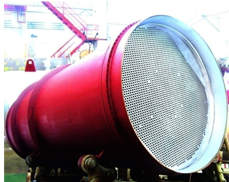
真空制盐一效加热室 Heating Chamber
